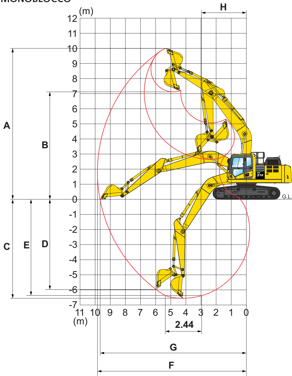
DIAGRAMMA DI SCAVO
